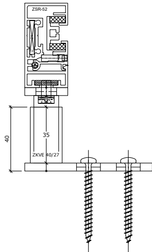
Halter ZKVE 40 / 27 -70
