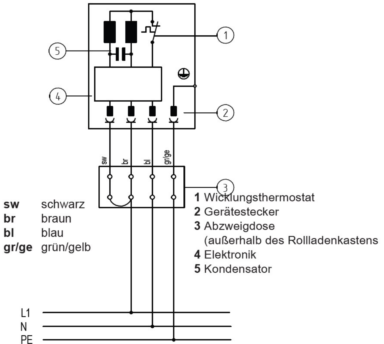
Anschlussbeispiel SunTop/Z M-868 RH 230 V / 50 Hz
