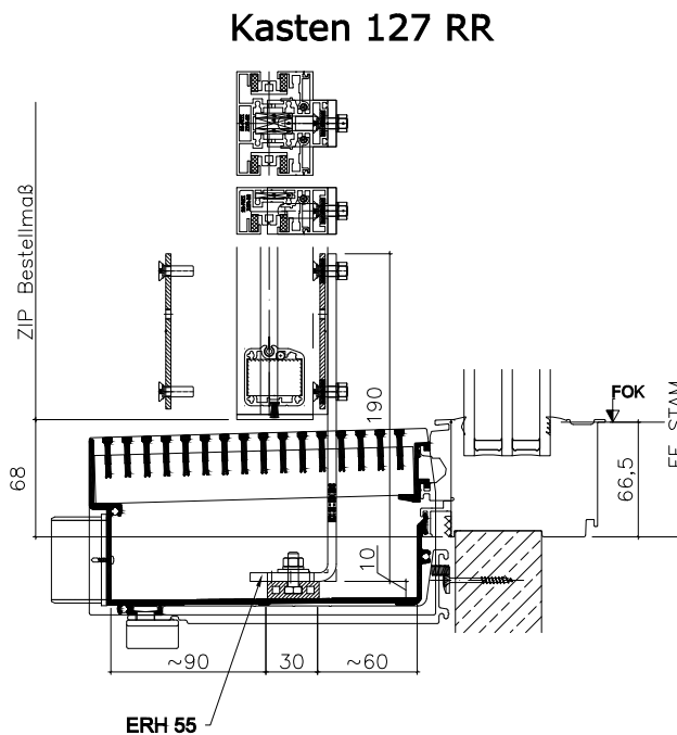
Kasten 127 RR mit ERH 55
