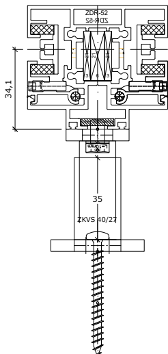
Halter ZKVS 40 / 27 -70
