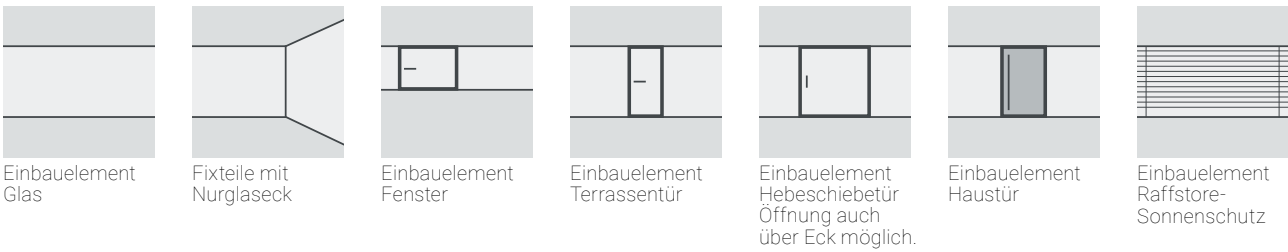
Einbauvarianten Ganzglassysteme
