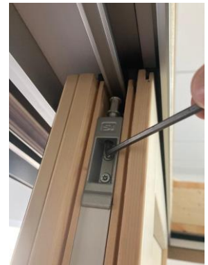
Führungsgleiter entfernen
