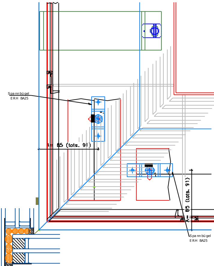
Abb. 20 System mit Entwässerungsschacht
