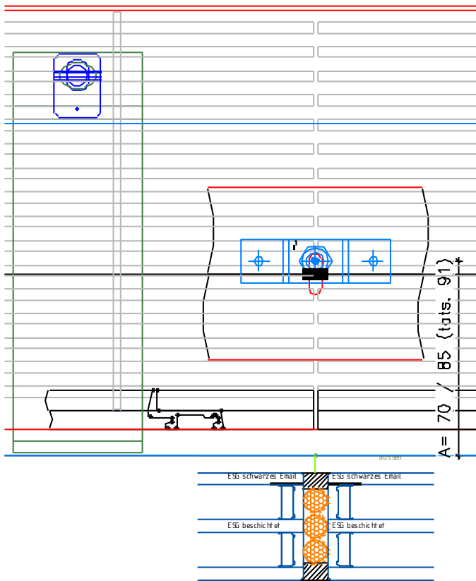
Abb. 17 System mit Entwässerungsschacht
