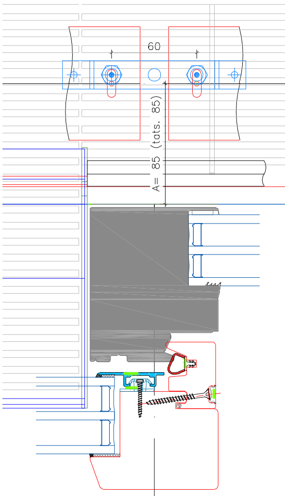
Abb. 16 System mit Entwässerungsschacht
