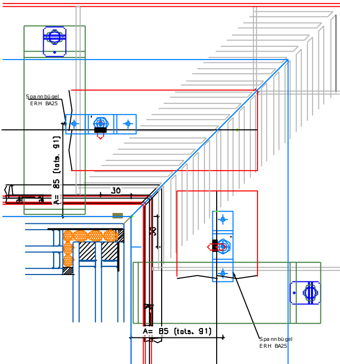
Abb. 19 System mit Entwässerungsschacht
