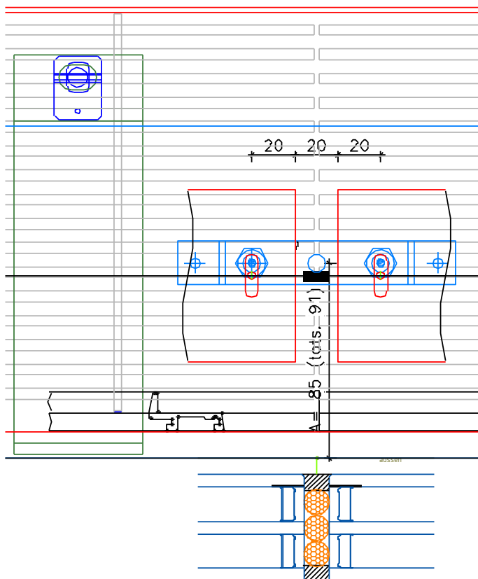
Abb. 18 System mit Entwässerungsschacht
