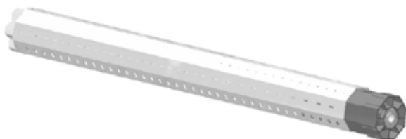
Zugeschnittene Welle mit Motor, Walzenkapsel mit Stahllager
