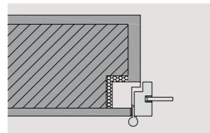
außenöffnend
