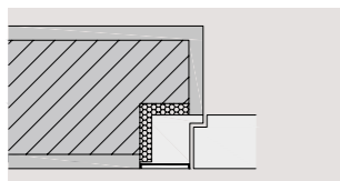
außenöffnend, bündig
