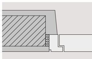
innenöffnend
