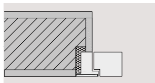
innenöffnend, bündig
