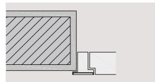
innenöffnend, versetzt
