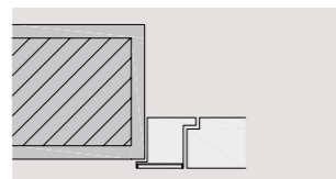
außenöffnend, versetzt
