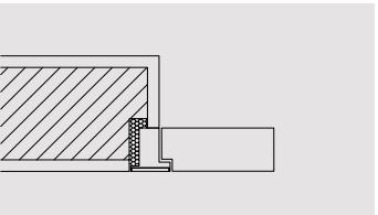
innen öffnend, bündig
