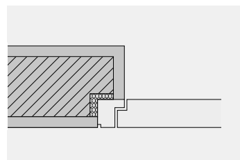
MET 40 innen und außen öffnend
